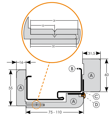
А) покрытие (корпус) коробки С) угловой наличник из алюминия Б) металлическая коробка D) прокладка
